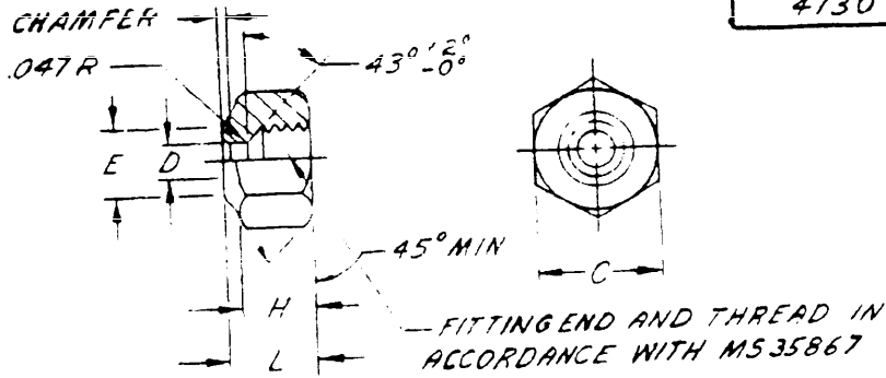
FLARE NUT
